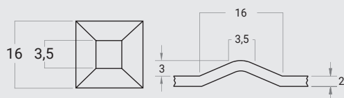
Detalle Repujado estándar de peldaños y mesetas
