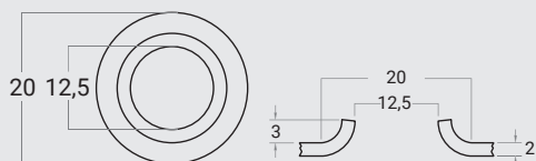
Detalle Perforado estándar de peldaños y mesetas
