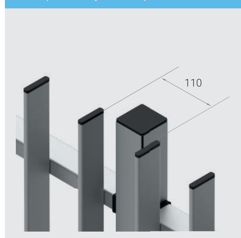
Detalle paño 50.10 y unión con pilar
