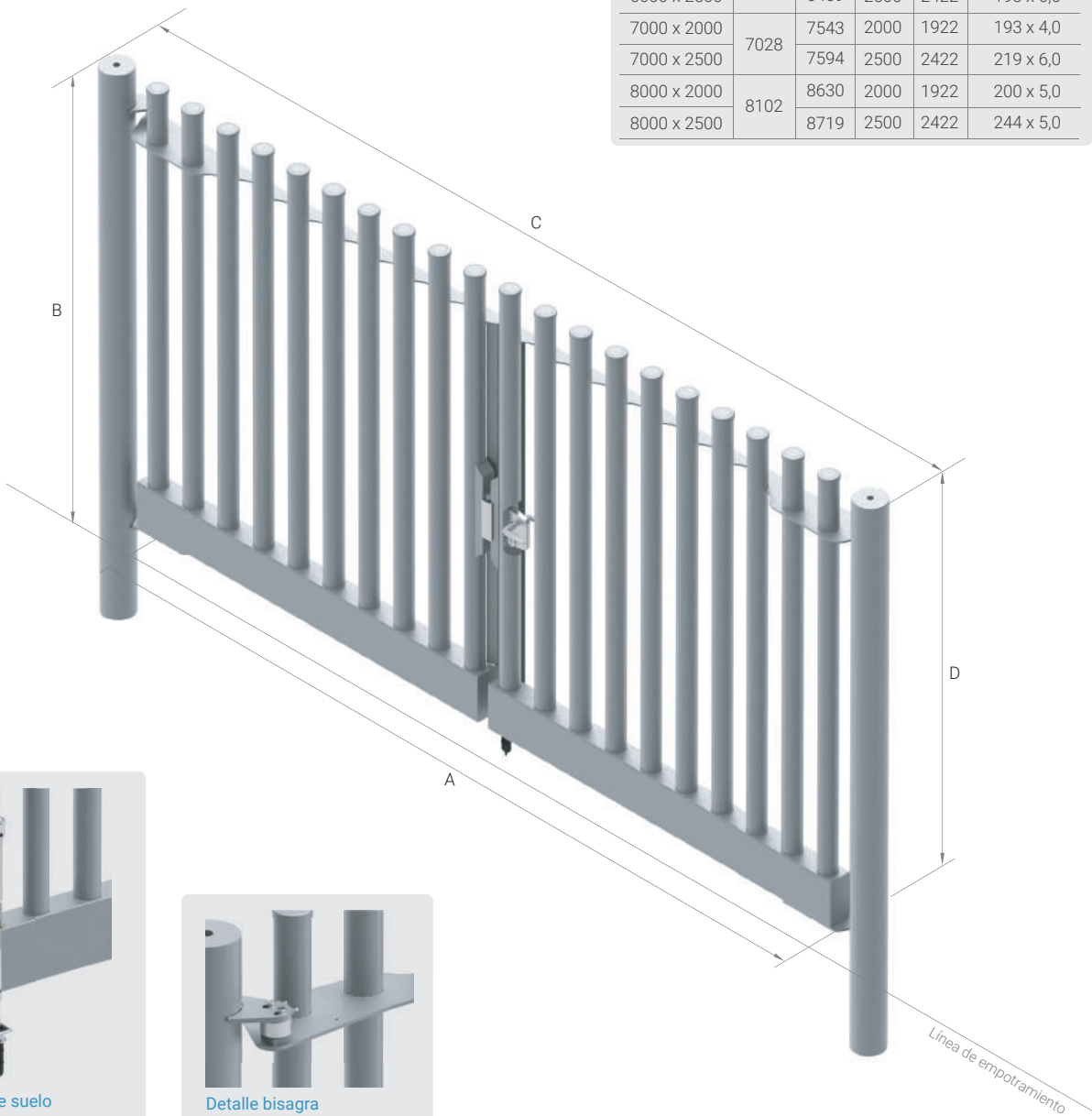
Detalle pestillo de suelo Pestillo y tope de suelo LOCINOX
