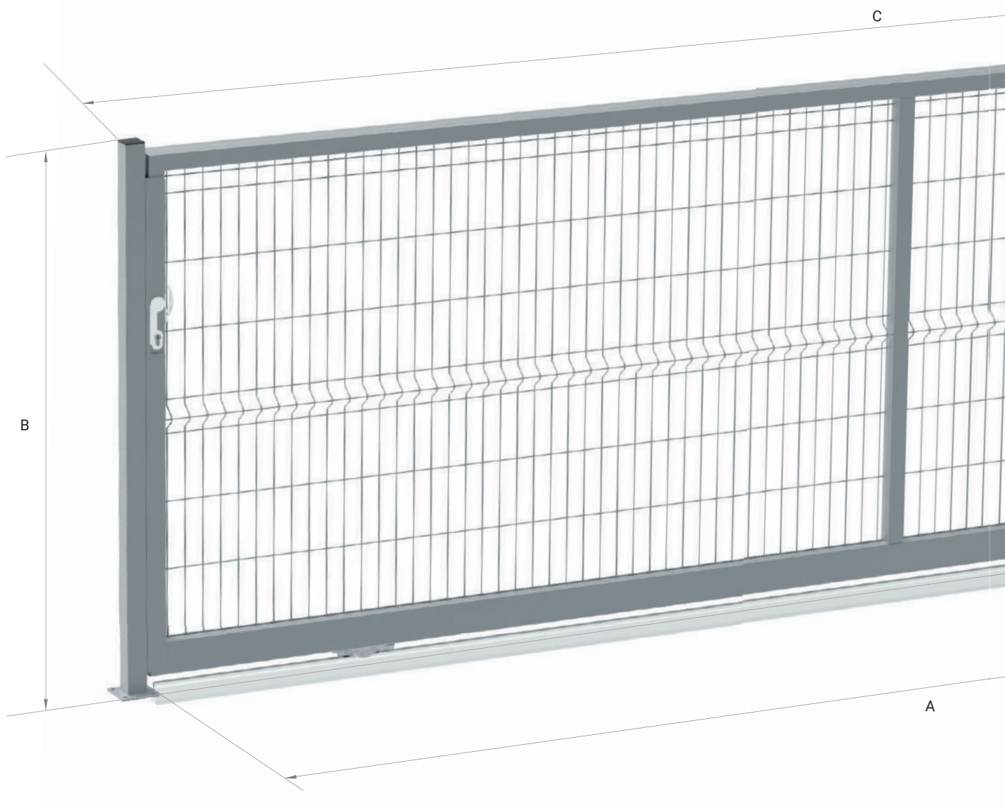
Detalle y pilar tope Pilar tope con perfil recepción
