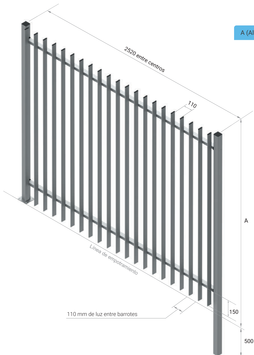
Detalle paño 50.10
