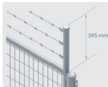
Detalle bayoneta Bayoneta alambre espino
