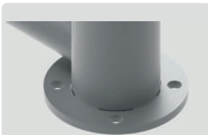
Detalle placa de anclaje Placa Ø 130 x 8 mm
