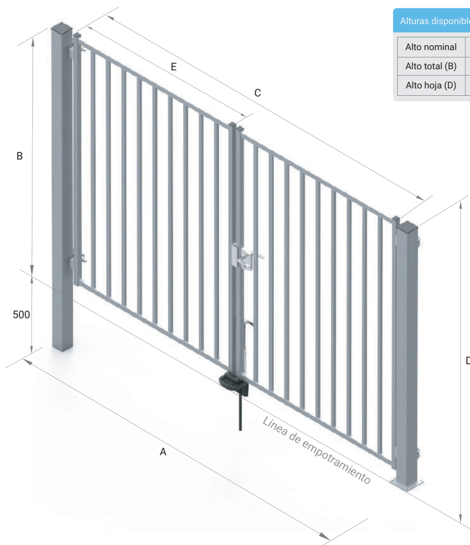
Ancho disponible puerta 2 hojas STYLE y TITAN FR14
