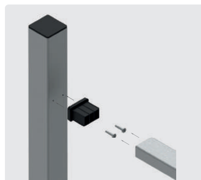
Detalle fijación
