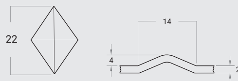
Detalle Repujado bajo pedido de peldaños y mesetas
