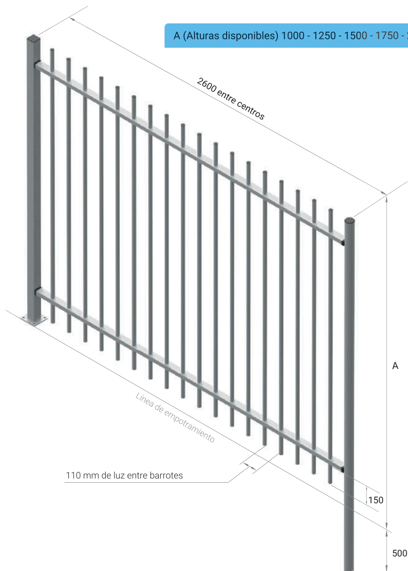
Detalle paño con barrote Ø 25 mm inglete
