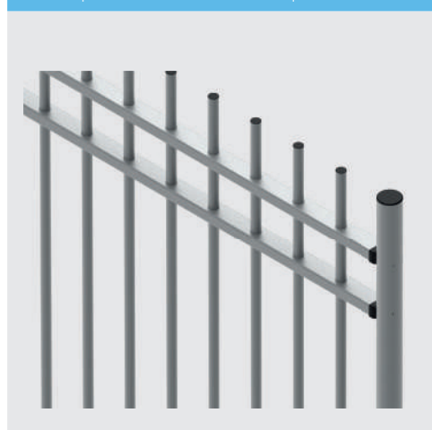
Detalle paño con doble travesaño superior sin soldadura
