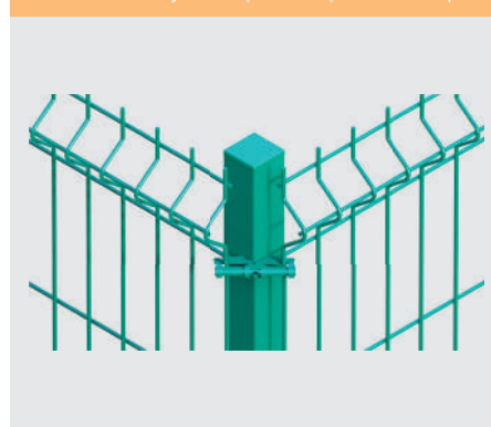
Detalle de montaje en esquina con poste Noumaplex
