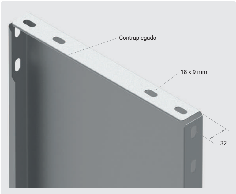
Información medidas bandejas
