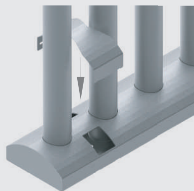
Paño EXPO atornillar arranque Detalle paño EXPO arranque y tapajuntas
