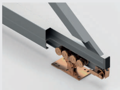
Detalle carro y rueda fin de curso Detalle carros y rueda en el interior de la guía.
