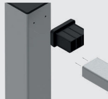
Detalle fijación Detalle fijación a poste cuadrado 60 x 60 mm
