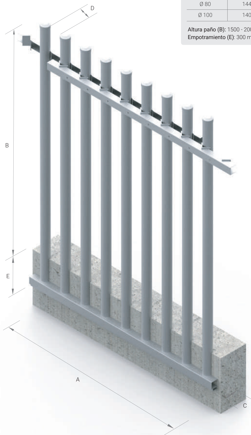
Paño EXPO balaustres sueltos Detalle plantilla empotrar
