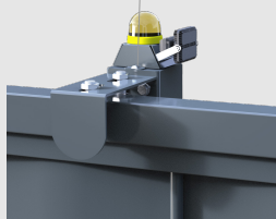
Detalle pilar guía Pletina oliva en pilar guía
