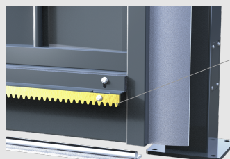
Detalle cremallera Detalle sujecion cremallera
