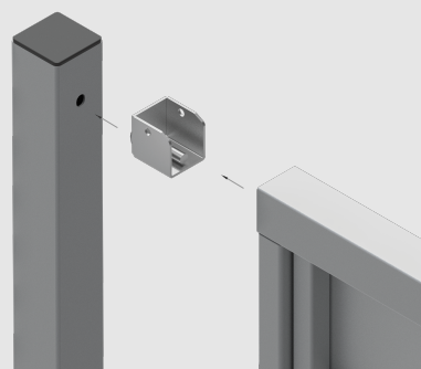
Detalle sistema de unión Unión mediante soporte FR14 50x50
